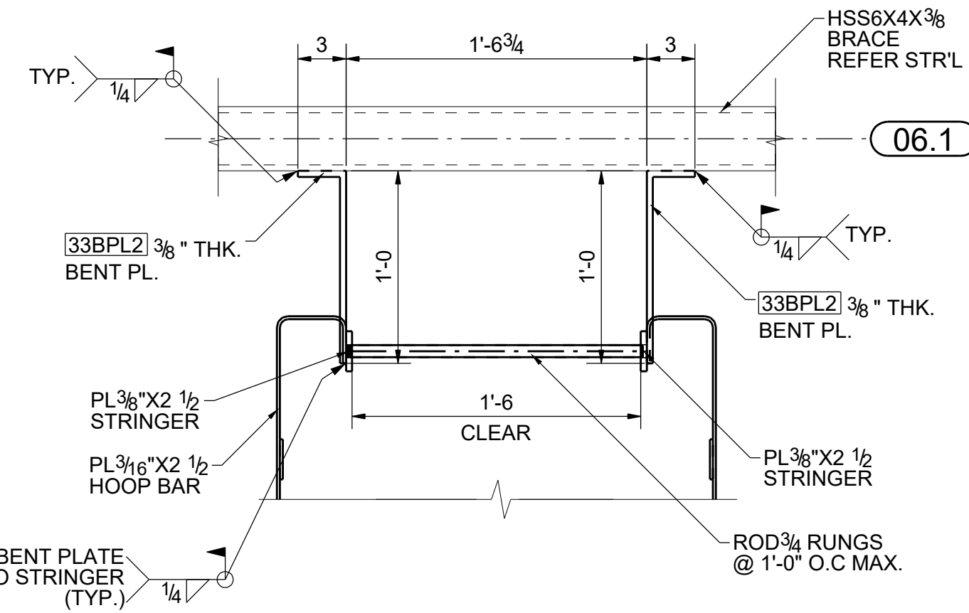
SECTION 6 - 6 33-E3301
